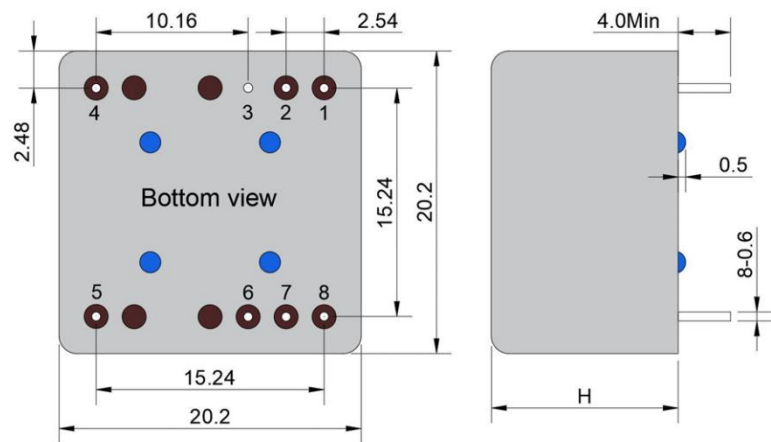
H=13mm,底部绝缘子高度 0.5mm,总高度 13.5mm
