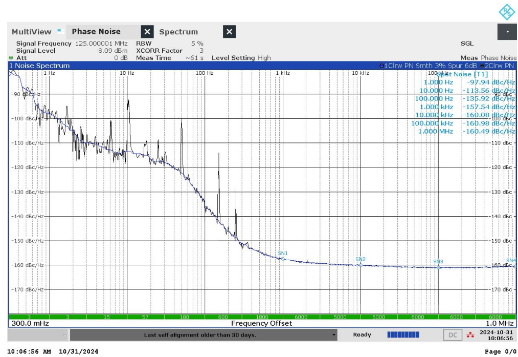
125MHz 相位噪声测试图
