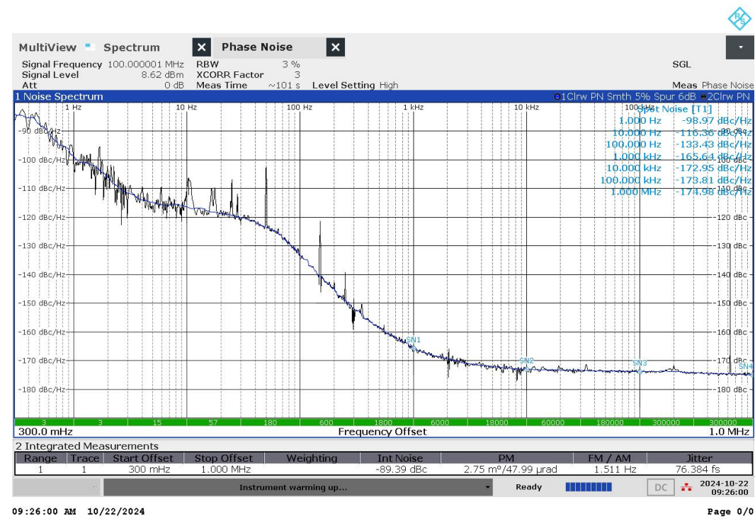
100MHz 相位噪声测试图
