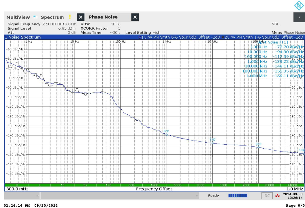
2500MHz 相位噪声测试图
