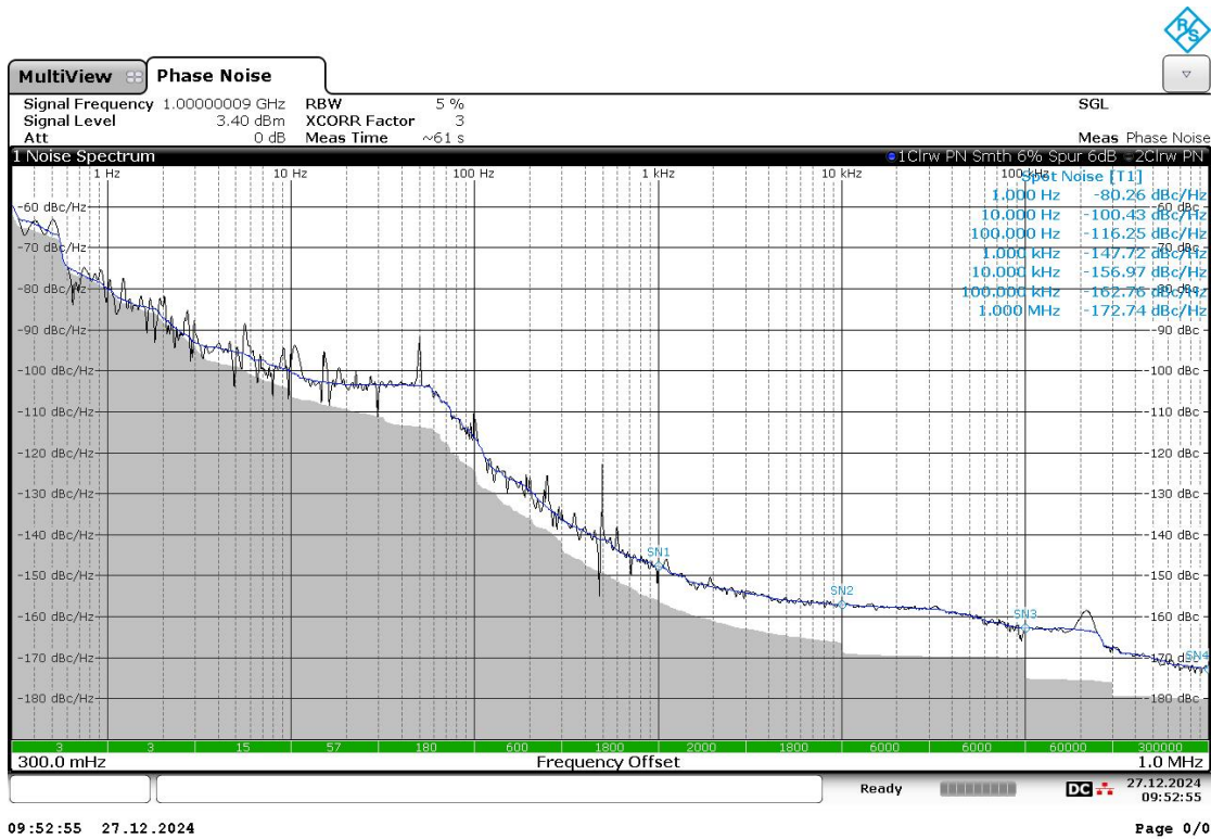
1000MHz 相位噪声测试图
