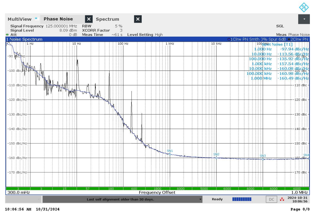
125MHz 相位噪声测试图
