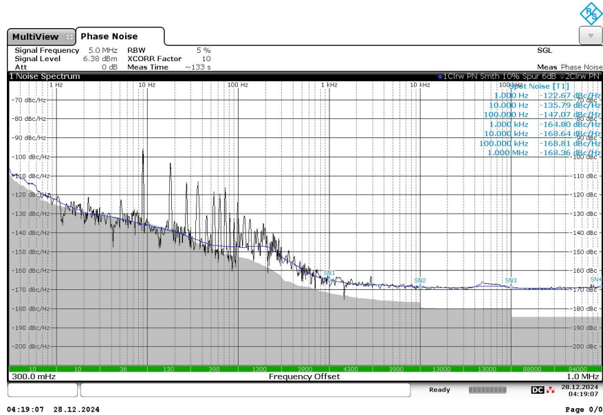
5MHz 相位噪声测试图
