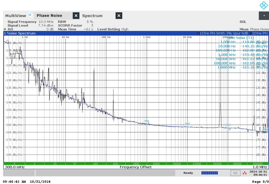
10MHz 稳定度测试图
