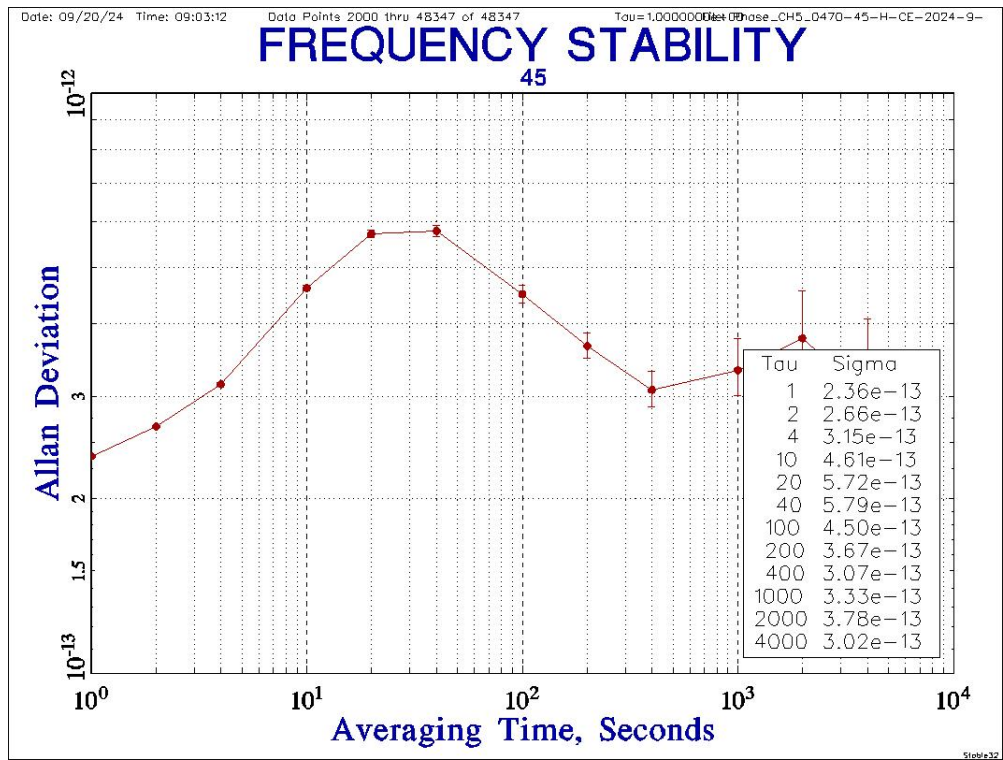
10MHz 稳定度测试图
