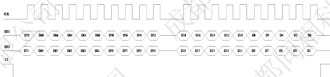
图 1 数据写时序图
